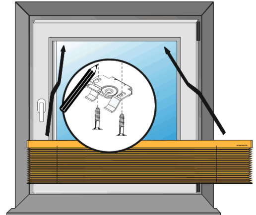
Halter mit Schwenkhebel
