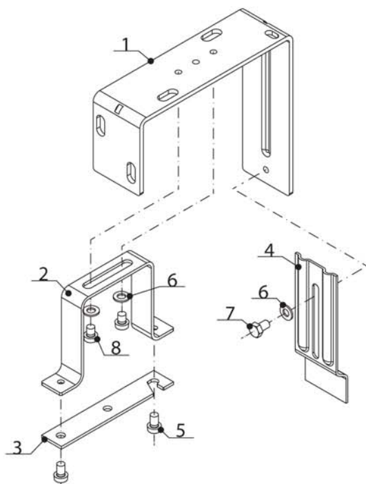
Montagebügel der Oberschiene Standard
