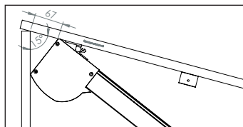
Montagehaken 15° Dachneigung
