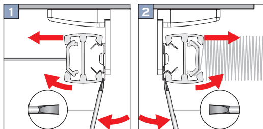
Winkelmontage Face fixing Montaż frontalny (nawierzchniowy) Монтаж на проем
