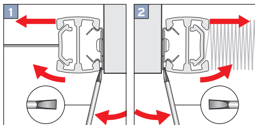
Falzmontage Top fixing Montaż w świetle szyby Монтаж в проем
