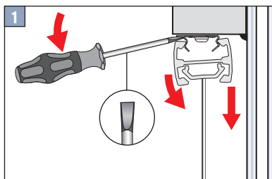
Falzmontage Top fixing Montaż w świetle szyby Монтаж в проем
