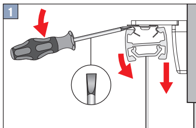
Winkelmontage Face fixing Montaż frontalny (nawierzchniowy) Монтаж на проем
